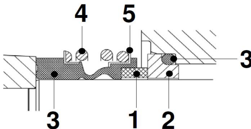
Риунок 3 – Схема торцового уплотнения
